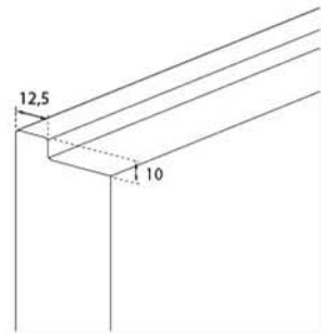
Avec recouvrement
