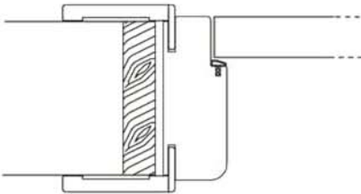
Forme du chambranle
