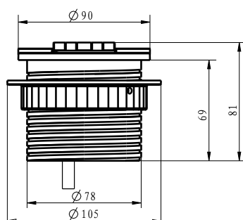
VUE LATÉRALE
