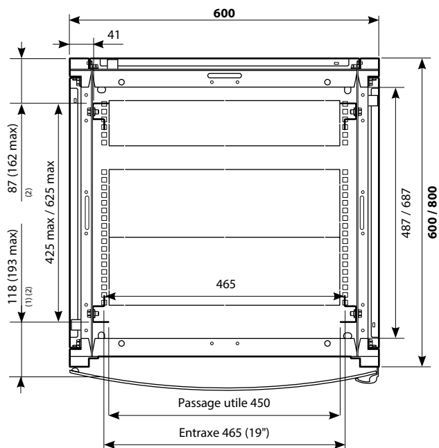
VUE EN COUPE A-A (3) (avec porte)
