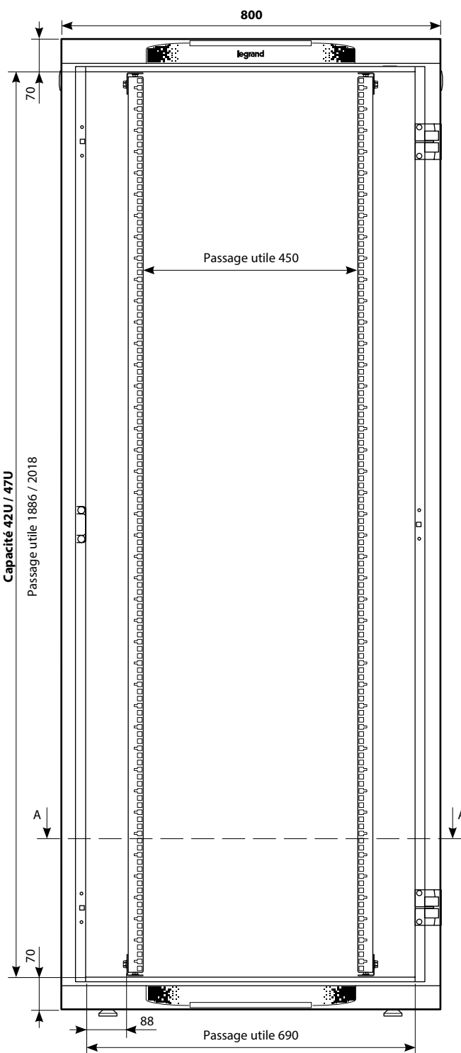
VUE DE FACE (sans porte)
