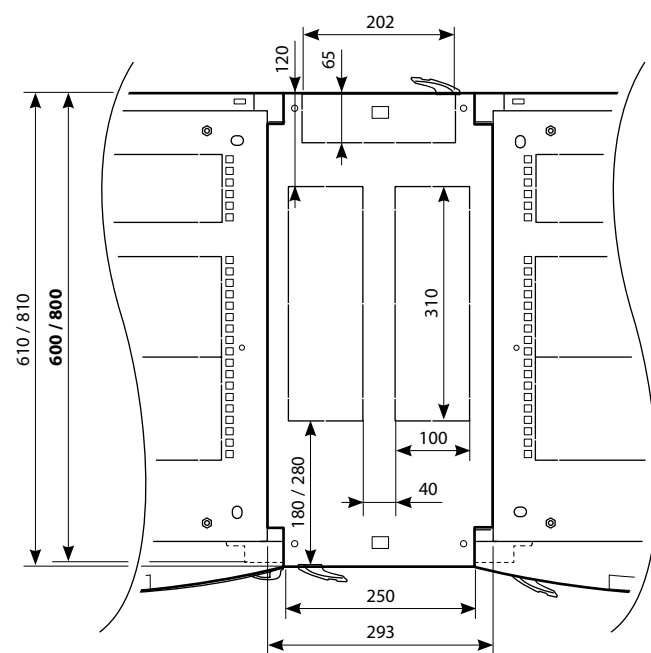
DÉTAIL VUE DE DESSUS
