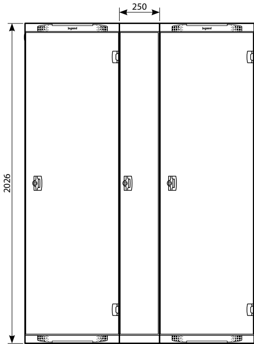
VUE AVANT
