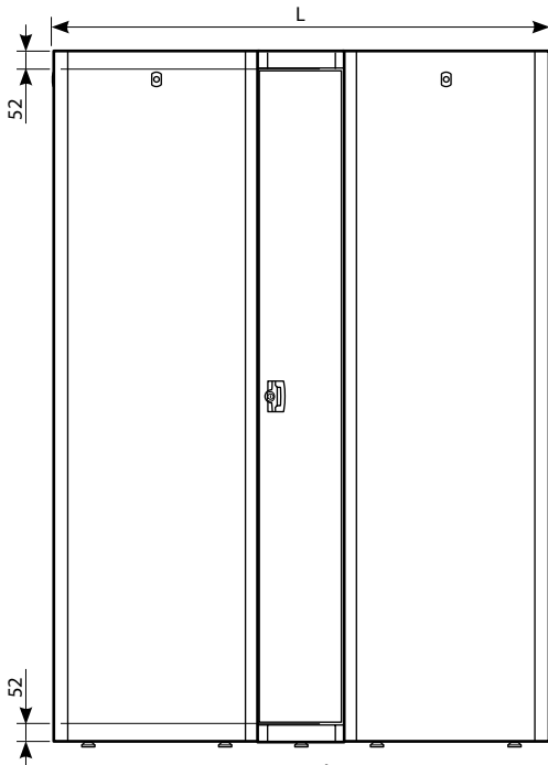
VUE ARRIÈRE
