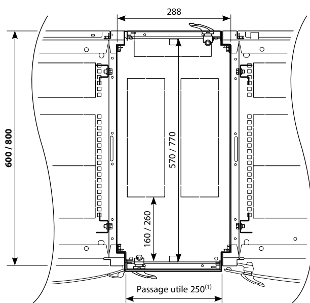
VUE INTÉRIEURE EN COUPE
