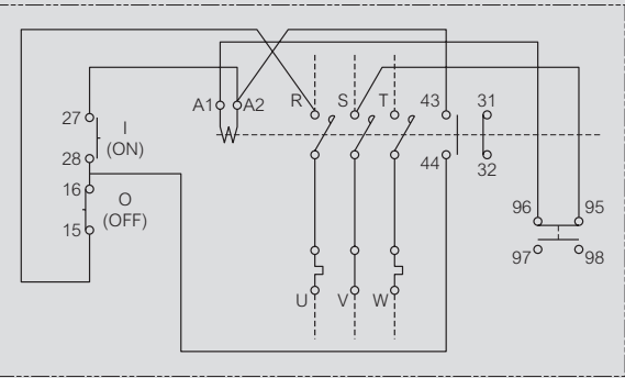
Schéma de câblage - Réf. 4 168 91
