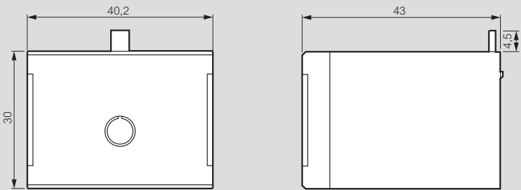
Retardé à l'ouverture - Réf. 4 168 70/71
