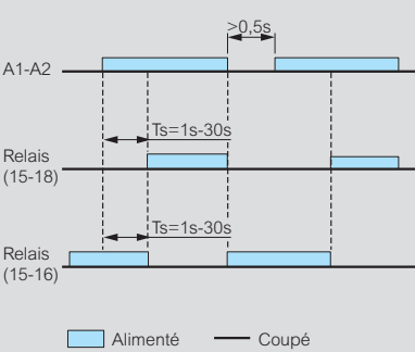
Retardé à l'ouverture - Réf. 4 168 70/71
