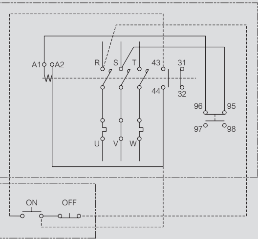
Schéma de câblage - Réf. 4 168 91
