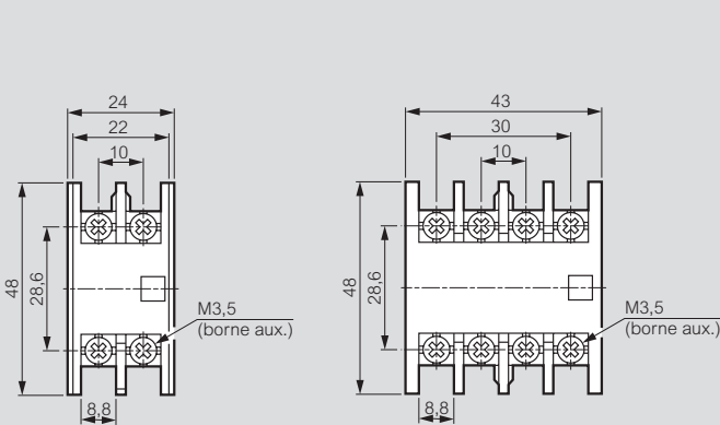
Montage frontal
