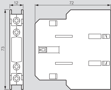
Montage latéral
