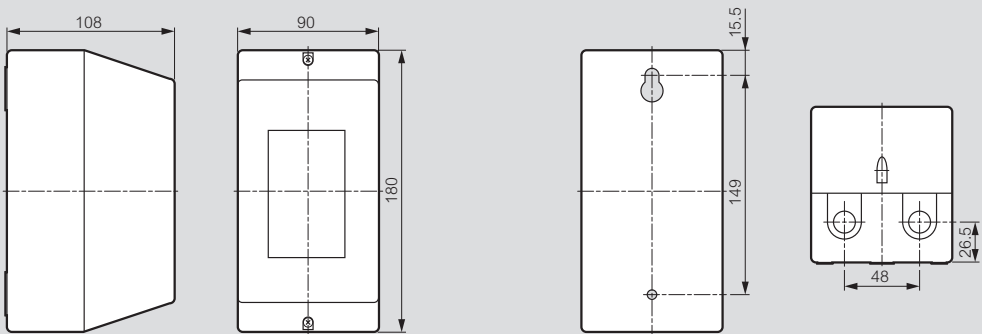
Sans bouton de commande - Réf. 4 168 90
