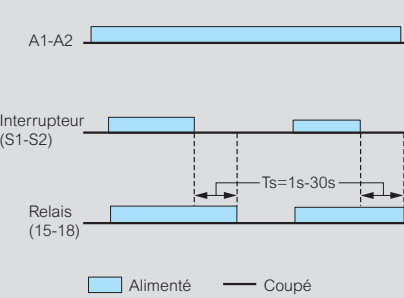
Retardé à la fermeture - Réf. 4 168 72/73
