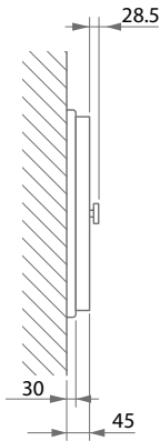
Flat door
