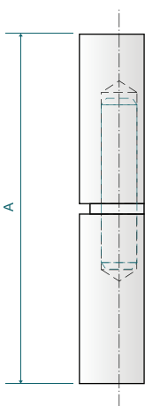
Paumelle à souder Goutte d'eau
