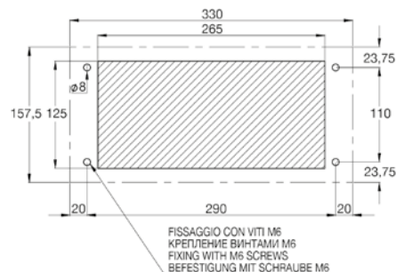
Dima di foratura (mm) Drilling pattern (mm)
