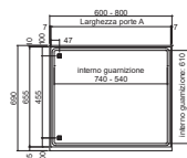
Visita frontale cassa 600 - 800
