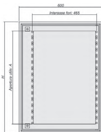
Vista fronte cassa con telaio rack 19"
