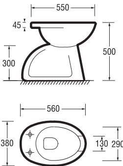
Cuvette simple sortie orientable pour personnes à mobilité réduite Washdown bowl orientable outlet 18 Kg
