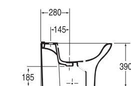
Bidet monotrou One hole bidet 22 Kg Réf. 111 410
