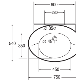
Colonne Pedestal 13 Kg Réf. 211 200
