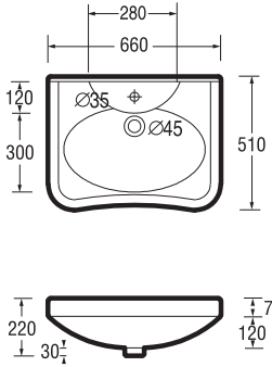
Lavabo pour personnes à mobilité réduite Washbasin 16 Kg
