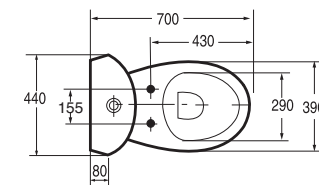
Cuvette simple sortie orientable Washdown bowl, orientable outlet 23 Kg Réf. 111 012
