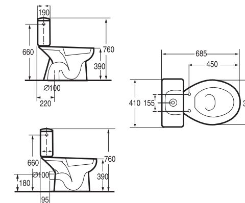
Cuvette monobloc sortie horizontale Close coupled WC, wall outlet 20 Kg Réf. 102 022
