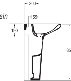
Semi colonne Half pedestal 8 Kg Réf. 211 240
