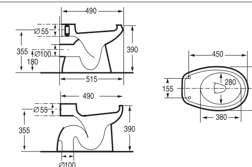
Cuvette simple sortie horizontale Washdown bowl, wall outlet 17 Kg Réf. 102 012
