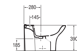
Bidet monotrou One hole bidet 22 Kg Réf. 111 410
