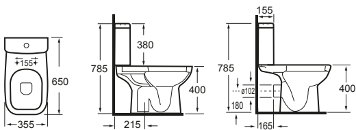
Réservoir / Cistern Réf. 101 112
