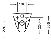
WC suspendu / Wall hung WC pan Réf. 101 032
