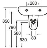
Semi colonne / Half pedestal Réf. 118 240
