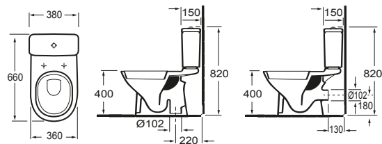
Réservoir / Cistern Réf. 118 112
