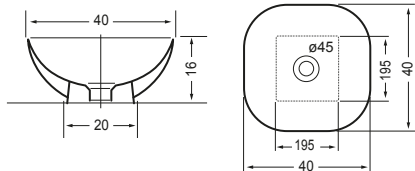
Vasque à poser Hand rinse basin Réf. 208 372
