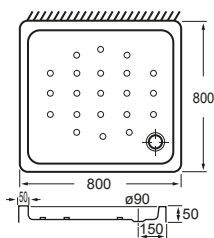
Receveur de douche carré à poser Squared shower tray raised Réf. 208 728
