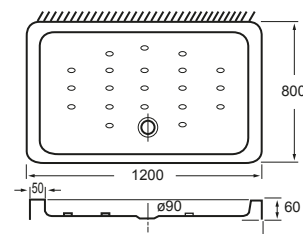
Receveur de douche Shower tray Réf. 208 727
