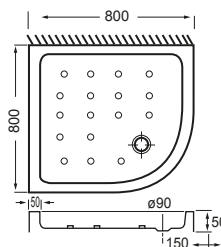
Receveur de douche angle à poser Corner shower tray raised Réf. 208 726
