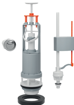
ENSEMBLE MÉCANISMES AVEC FLOTTEUR ALIMENTATION BASSE 61E5A00
