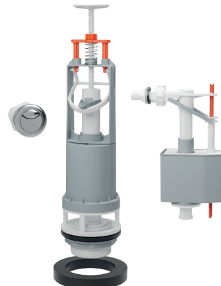
ENSEMBLE MÉCANISME DE CHASSE À BOUTON POUSSOIR AVEC FLOTTEUR COULISSANT 61AHA00
