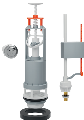
ENSEMBLE MÉCANISMES AVEC FLOTTEUR ALIMENTATION BASSE ET EMBOUT EN LAITON 61E6A00
